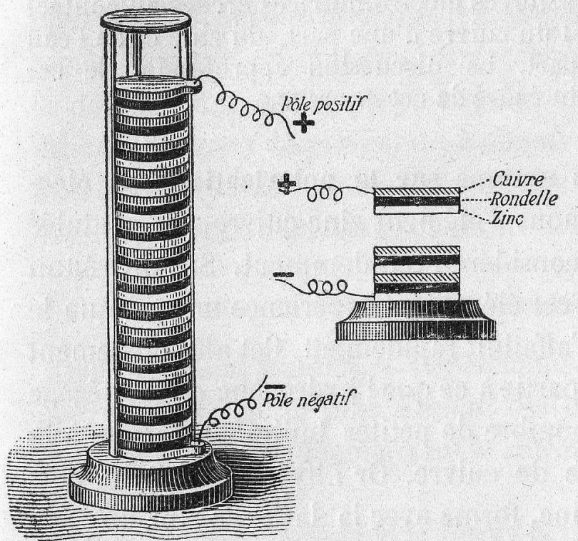
Fig. 283. — Pile de Volta.
